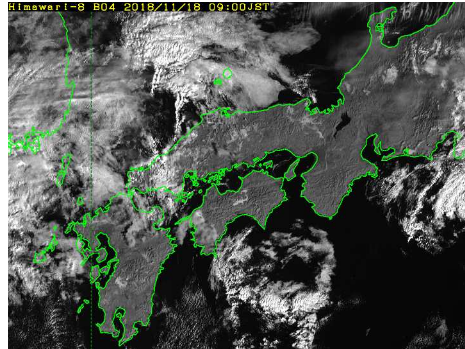
B04 ( 0.86 \mu\text{m} ) 近赤外画像
