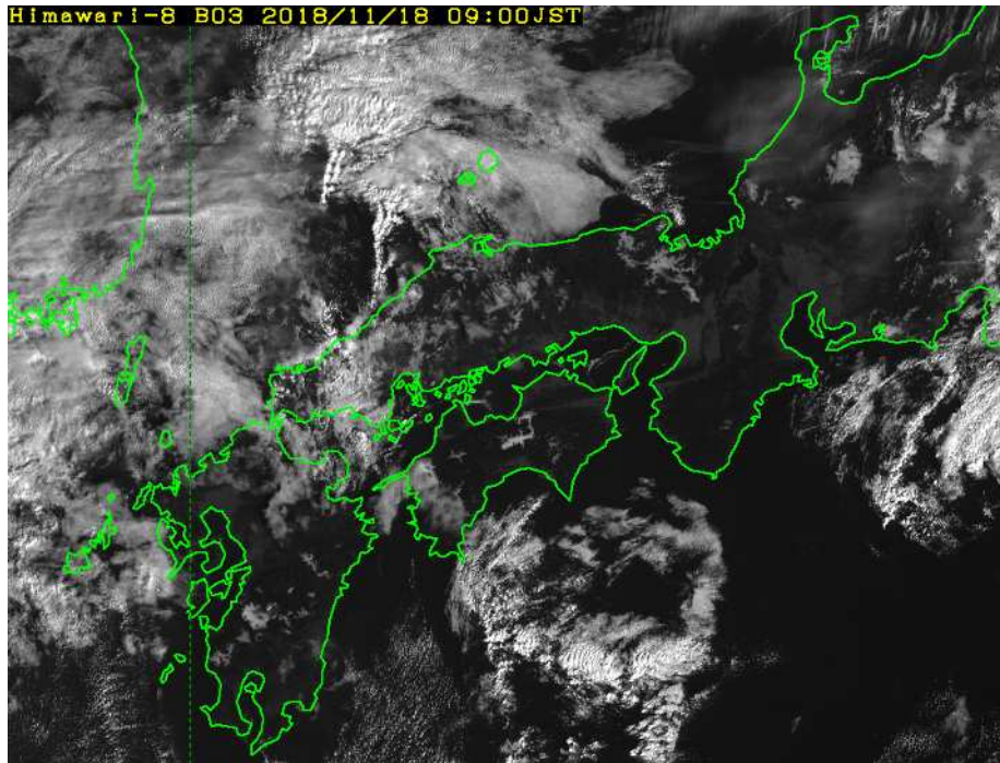
B03 ( 0.64 \mu\text{m} ) 可視画像
